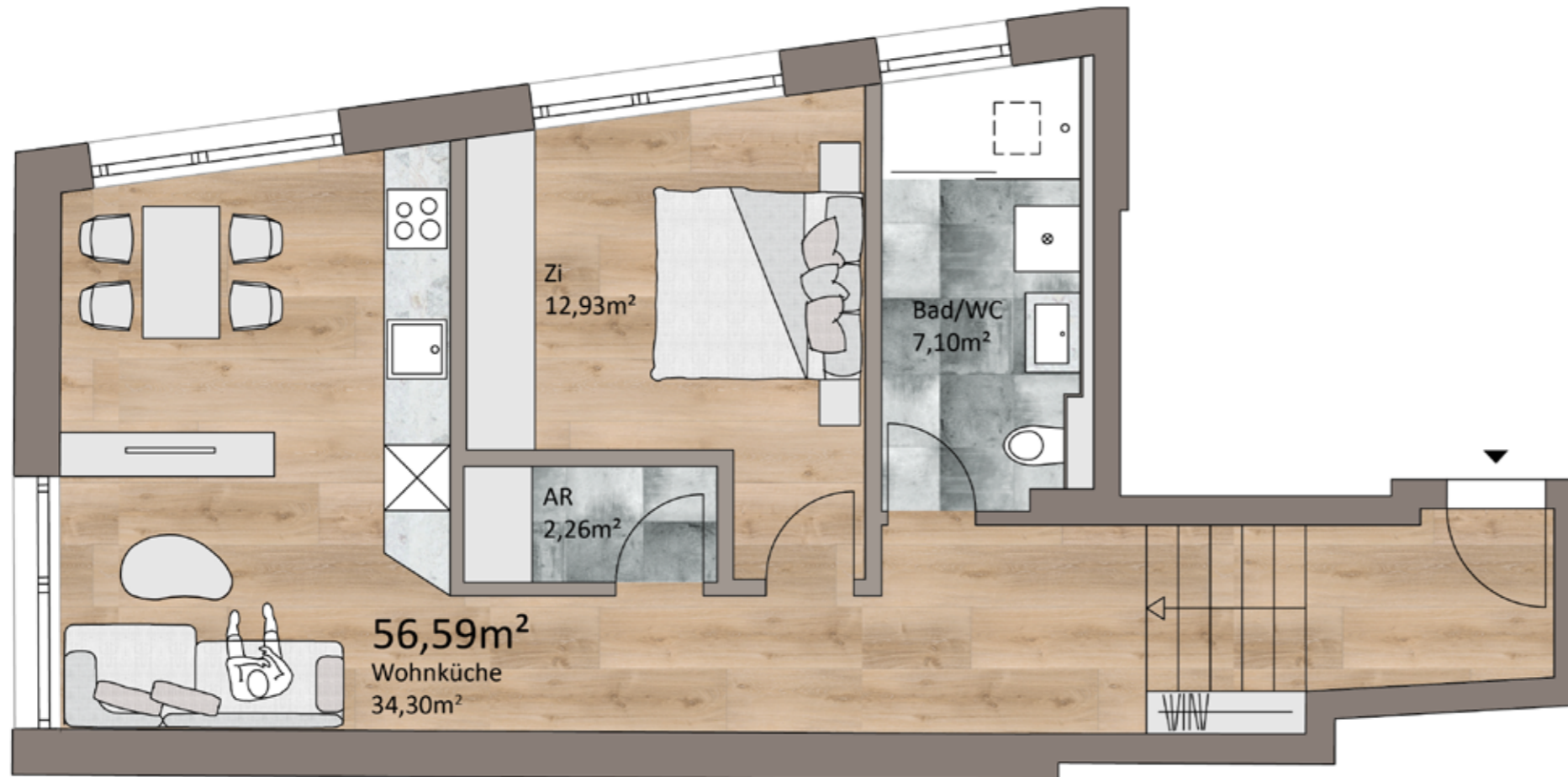
Grundriss TOP L01, Erdgeschoss
